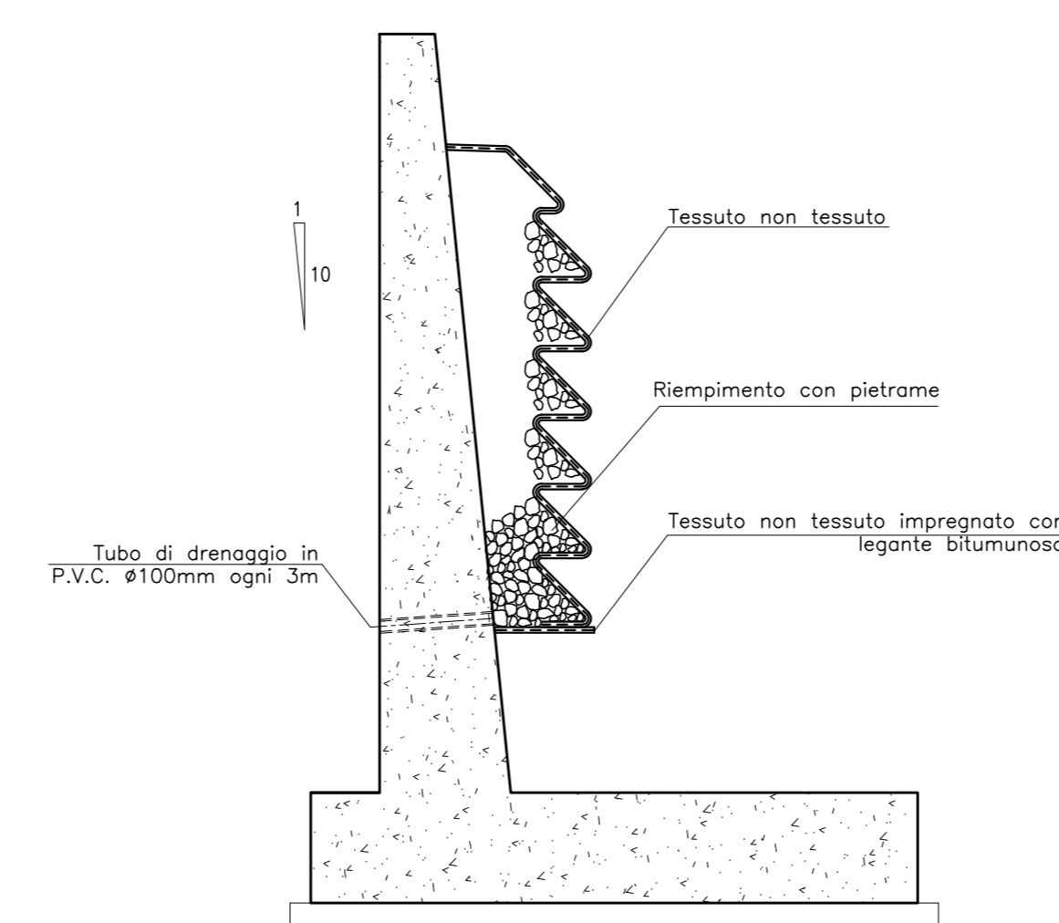
SEZIONE TIPO MURO DI SOSTEGNO SCALA 1:50
