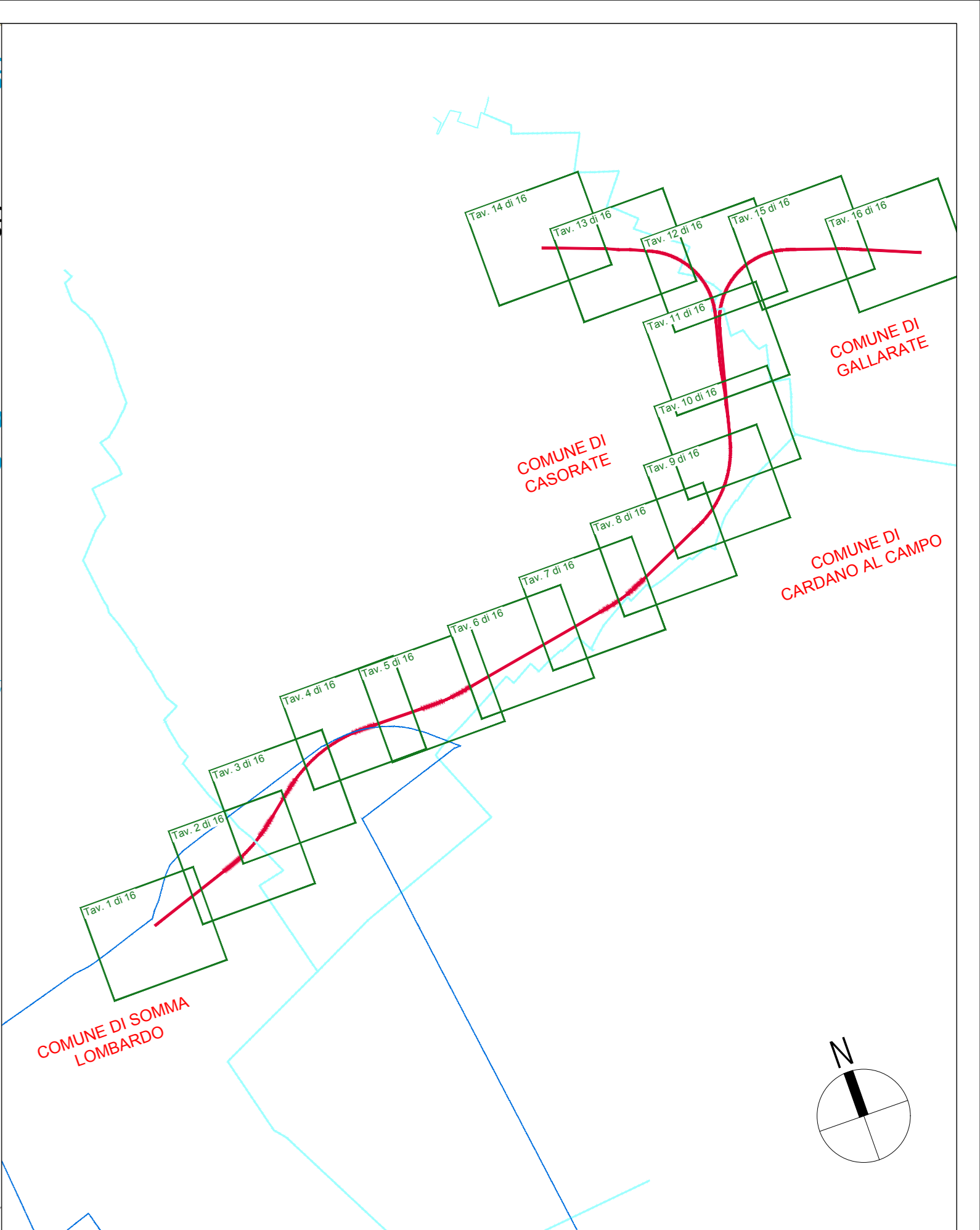
PLANIMETRIA DI PROGETTO SCALA 1:500
