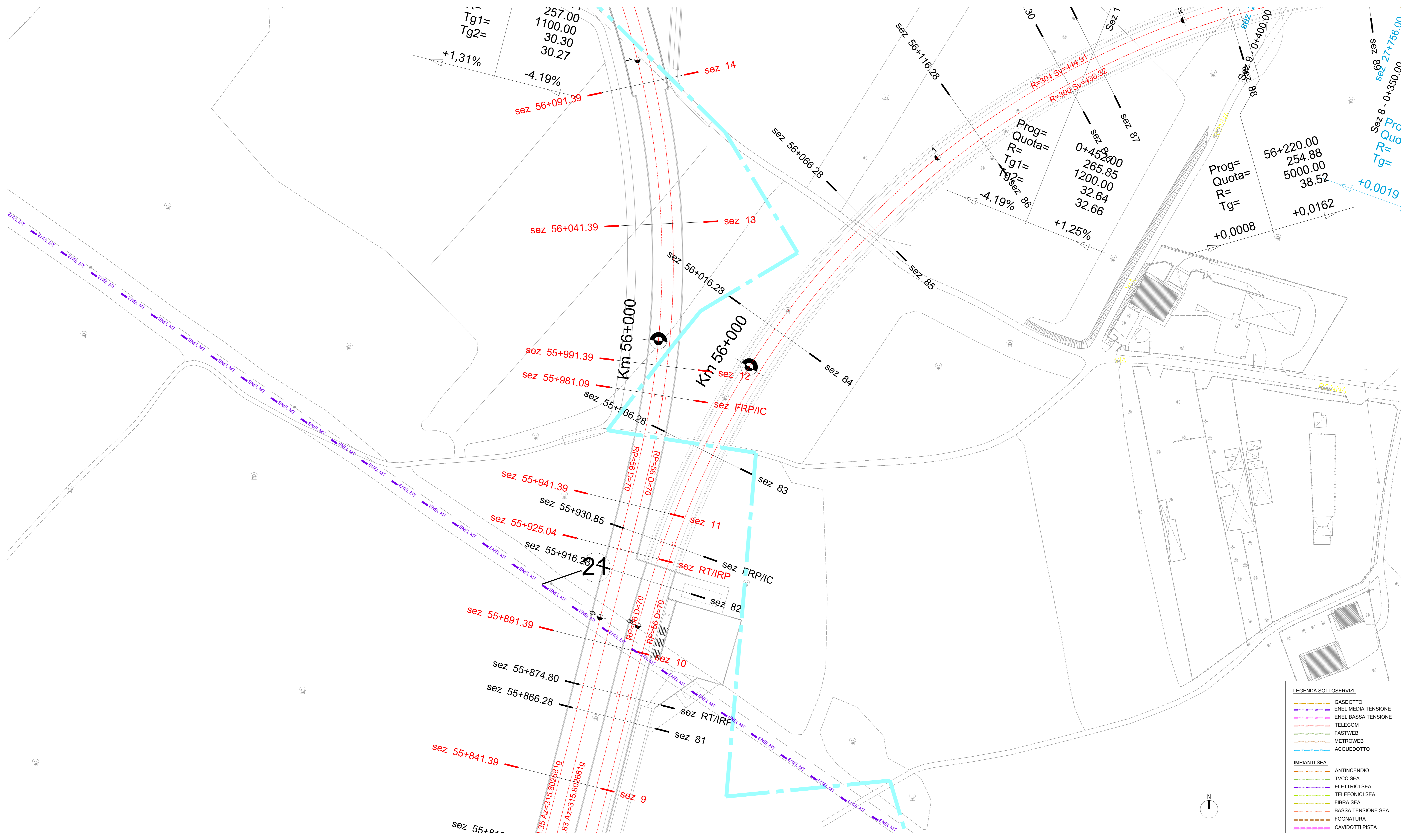
PLANIMETRIA DI PROGETTO SCALA 1:500
