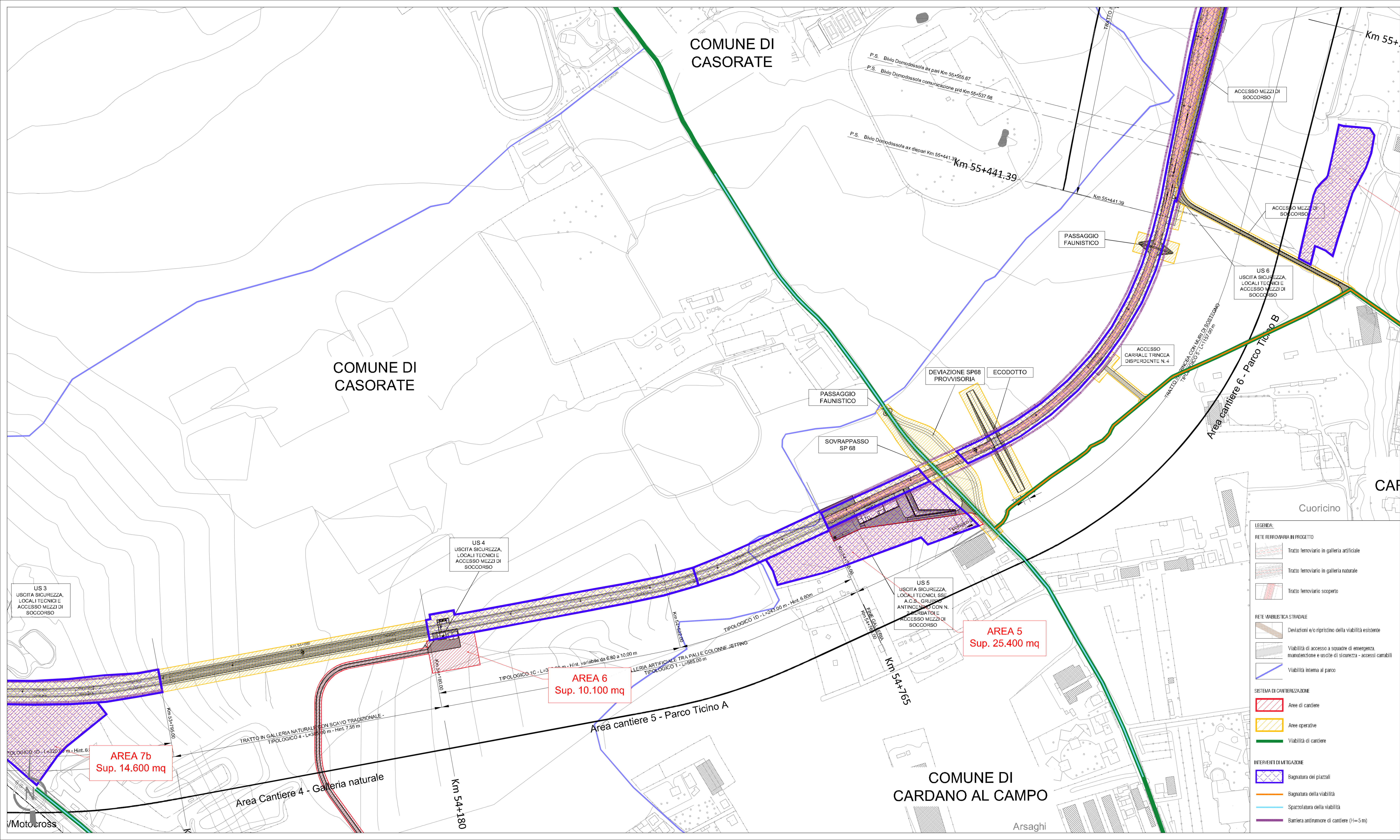
PLANIMETRIA DI PROGETTO SCALA 1:2.000 KEY-PLAN
